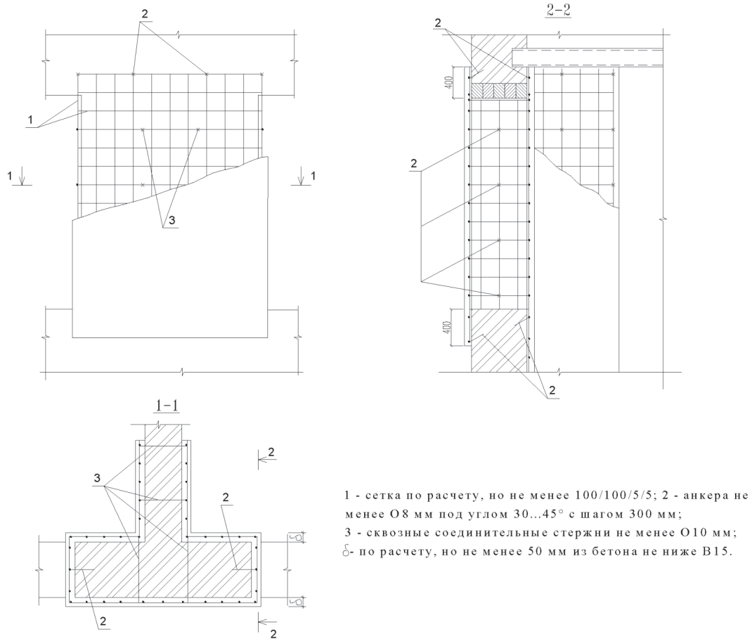
Рисунок В.13 – Усиление простенков, примыкающих к внутренним стенам
