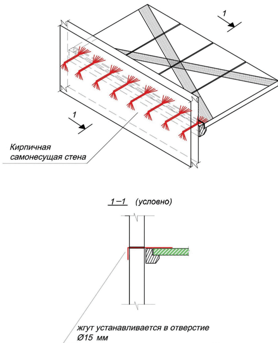
Рисунок В.34 – Создание единого диска перекрытия за счет системы внешнего армирования углеволокном
