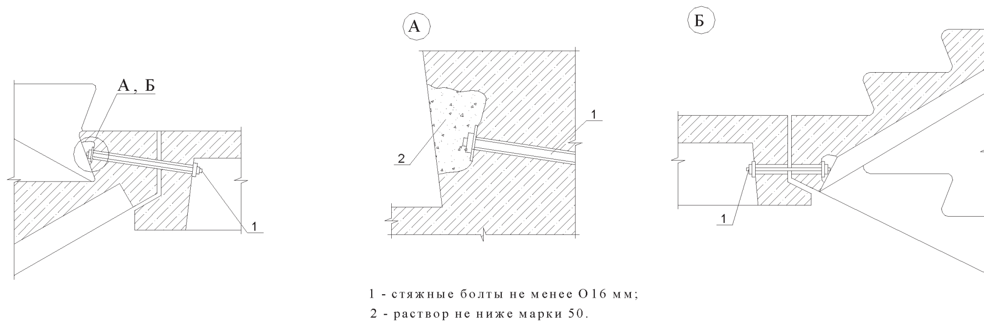
Рисунок В.20 – Анкеровка лестничных площадок
