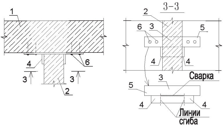
Рисунок В.25 – Узлы крепления перегородок к железобетонным перекрытиям и покрытиям
