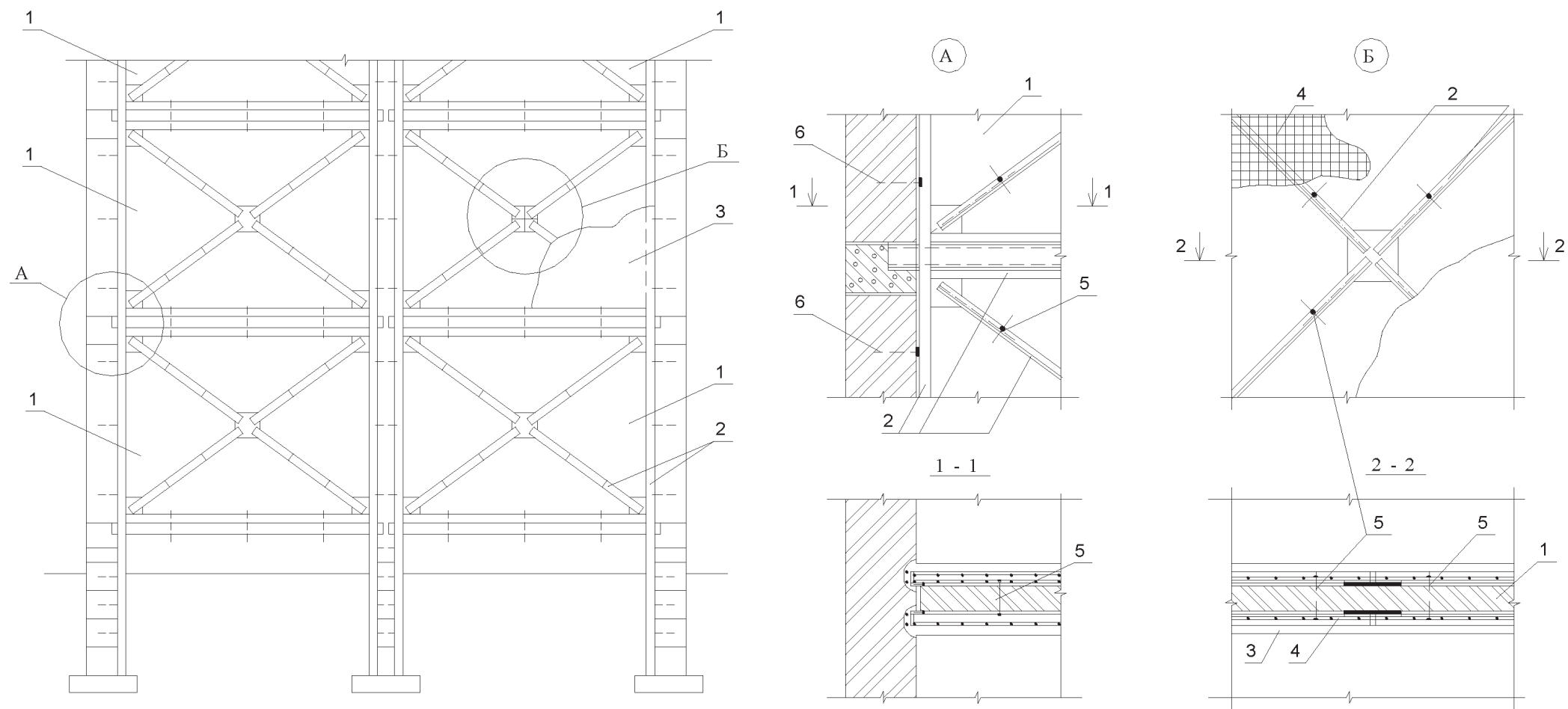
Рисунок В.9 – Преобразование кирпичной перегородки в диафрагму жесткости
