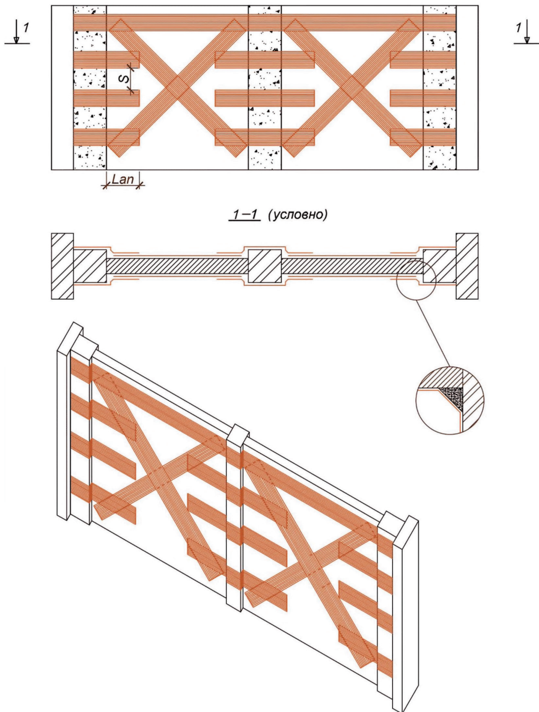
Рисунок В.42 – Усиление несущих кирпичных перегородок за счет системы внешнего армирования углеволокном (вариант 2)
