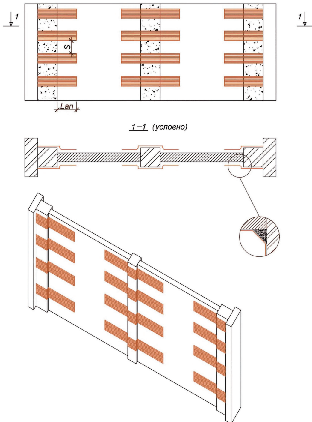
Рисунок В.44 – Усиление несущих железобетонных перегородок за счет системы внешнего армирования углеволокном (вариант 2)
