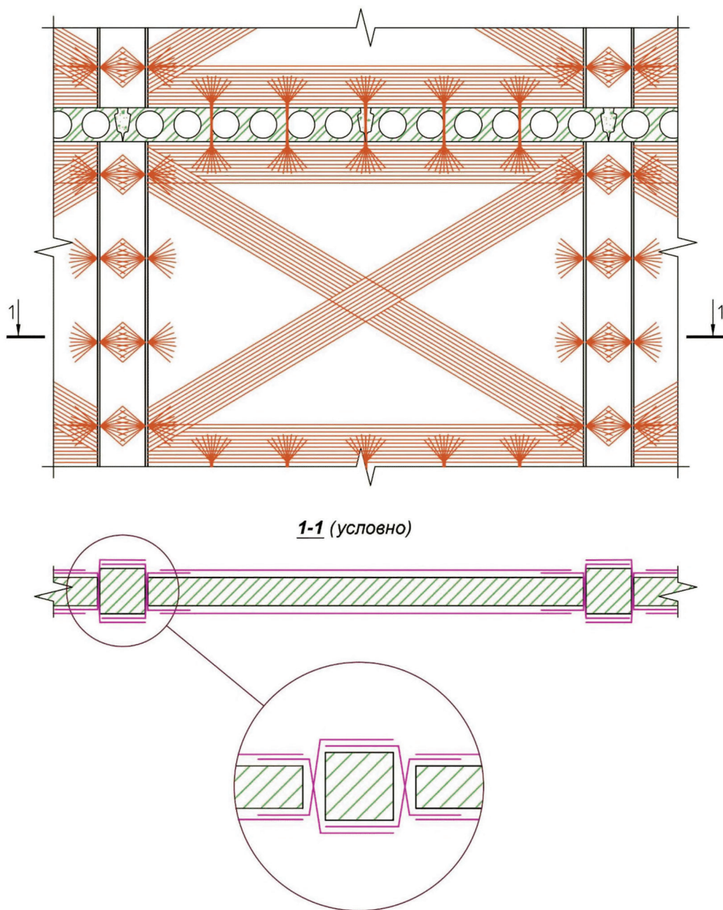
Рисунок В.38 – Создание диафрагм жесткости из каменных стен за счет системы внешнего армирования углеволокном
