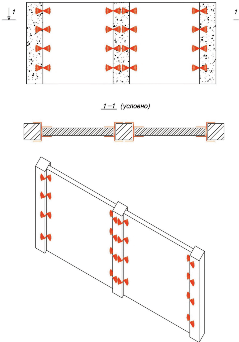
Рисунок В.43 – Усиление ненесущих железобетонных перегородок за счет системы внешнего армирования углеволокном (вариант 1)
