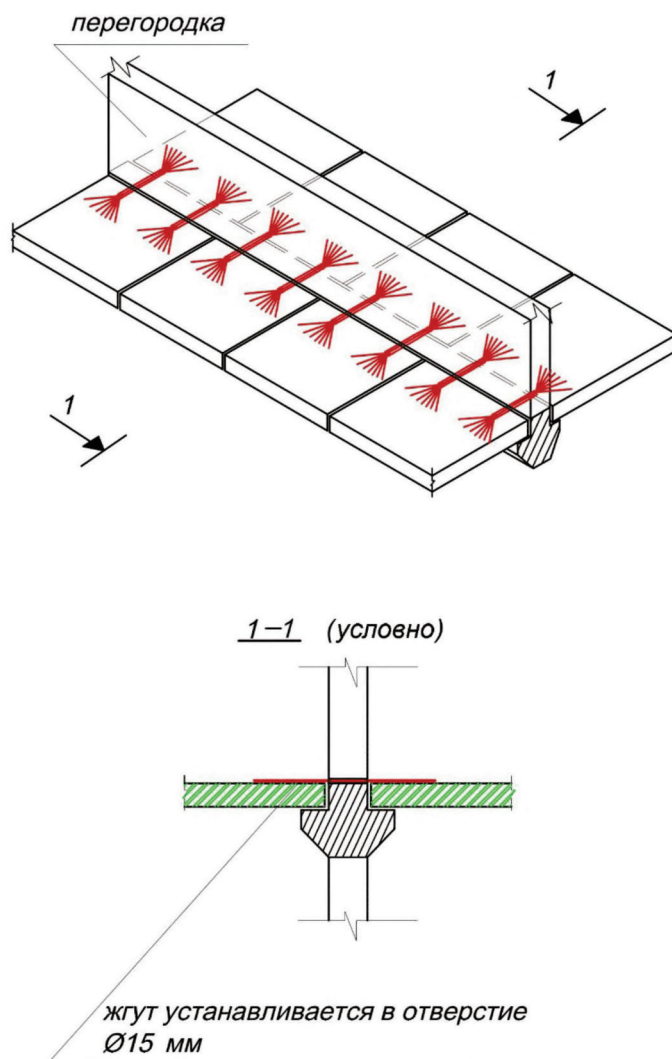
Рисунок В.35 – Создание единого диска перекрытия за счет системы внешнего армирования углеволокном
