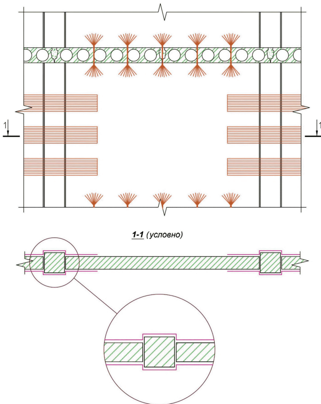
Рисунок В.39 – Создание диафрагм жесткости из железобетонных стен за счет системы внешнего армирования углеволокном
