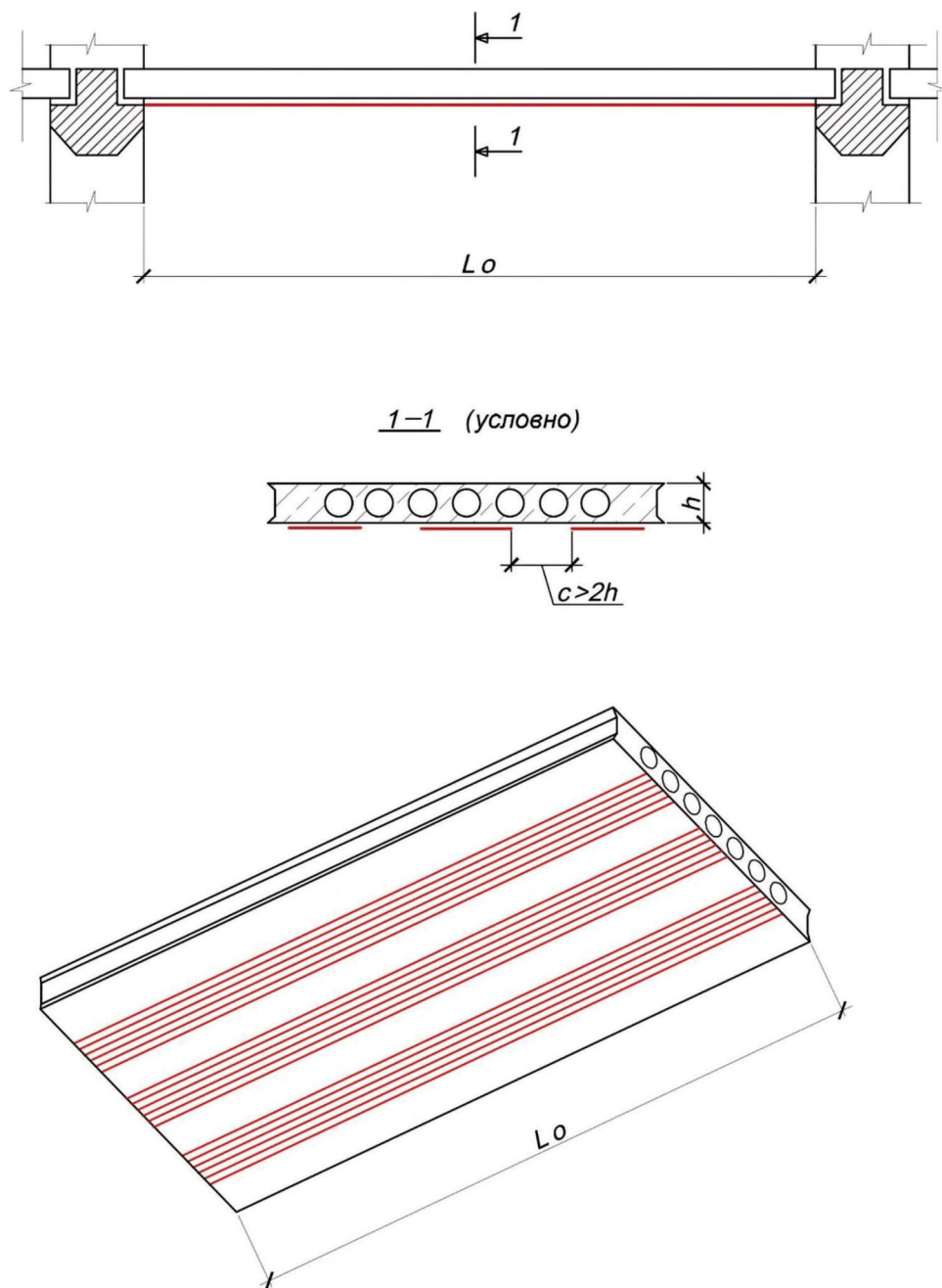
Рисунок В.32 – Усиление железобетонных плит перекрытия за счет системы внешнего армирования углеволокном. Повышение прочности пустотных плит
