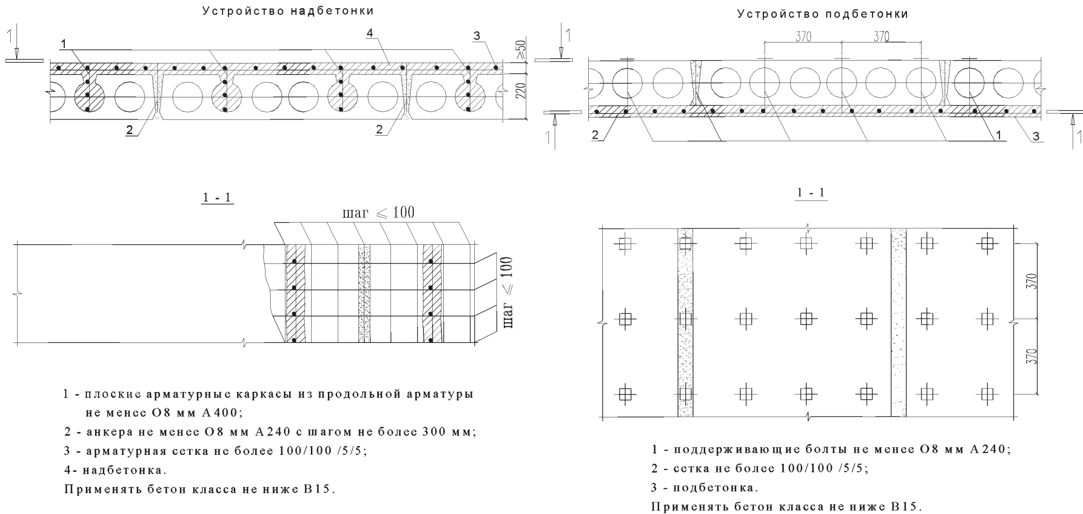
Рисунок В.1 – Усиление пустотных плит перекрытия
