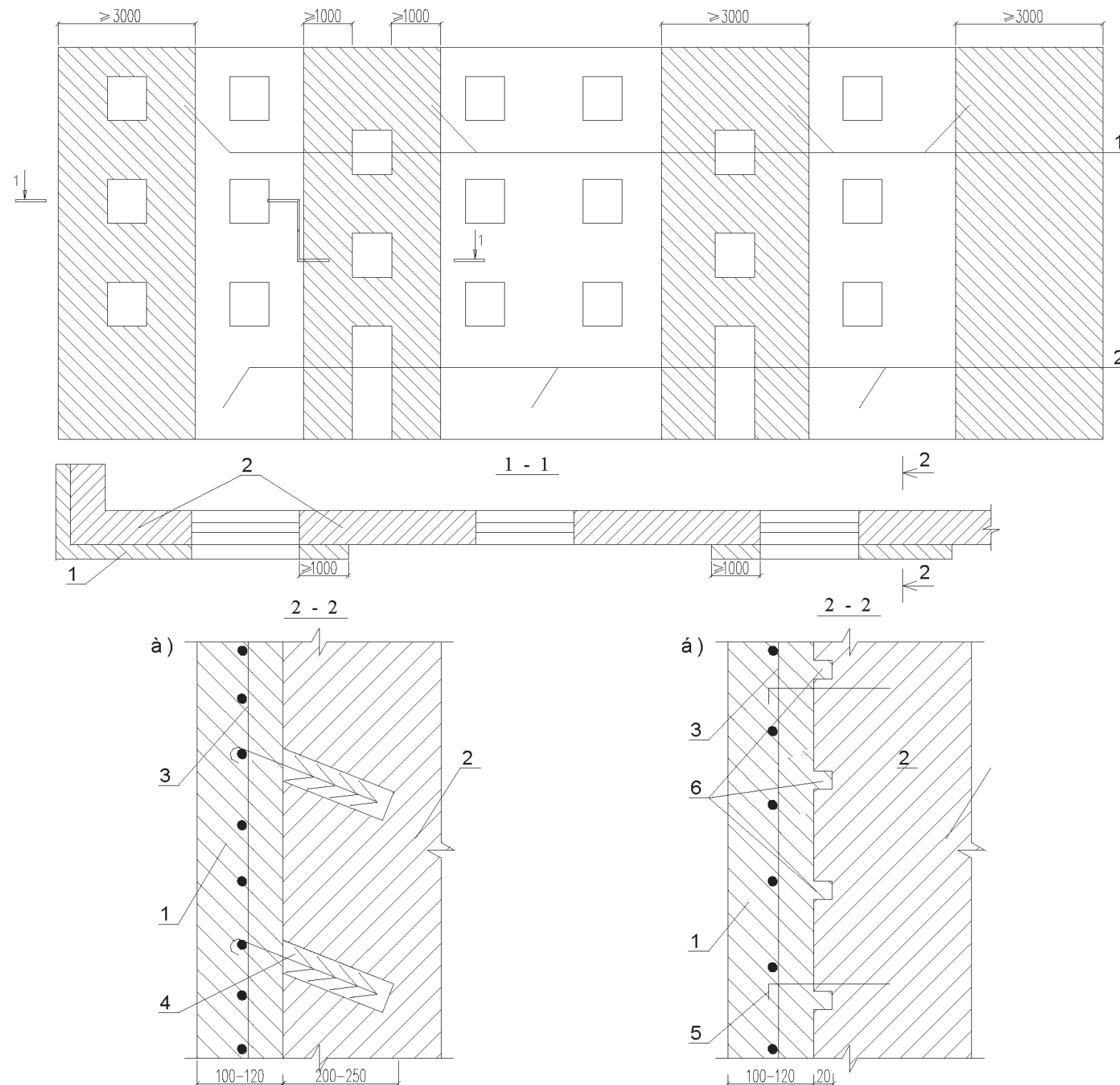
Рисунок В.4 – Устройство односторонних железобетонных аппликаций
