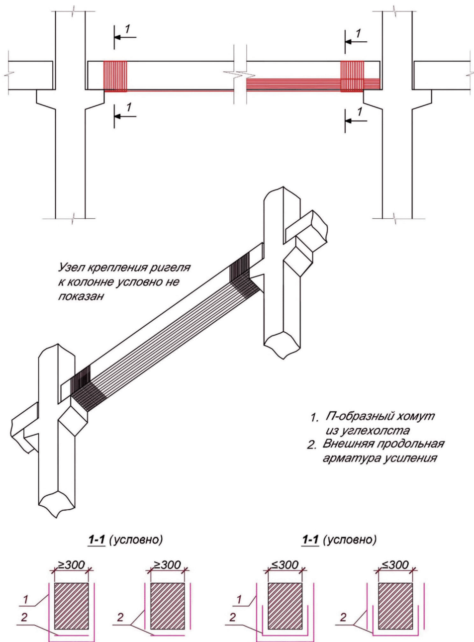
Рисунок В.30 – Усиление железобетонных ригелей за счет системы внешнего армирования углеволокном. Повышение прочности нормальных сечений
